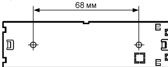
Рис.9 Присоединительные размеры
